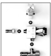
Magnetventil Mischung über DMK-Mischer zur Direktmontage auf Eckventil mit RüVe in KW/WW Eckventil(bauseitig)
